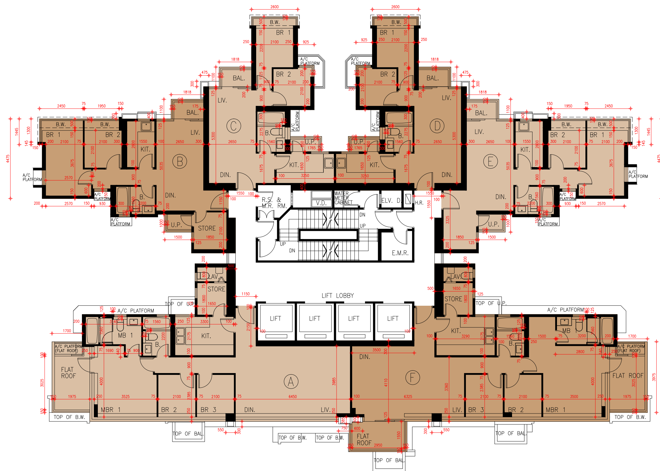
Tower 9 49/F Floor Plan 第9座49樓樓面平面圖
