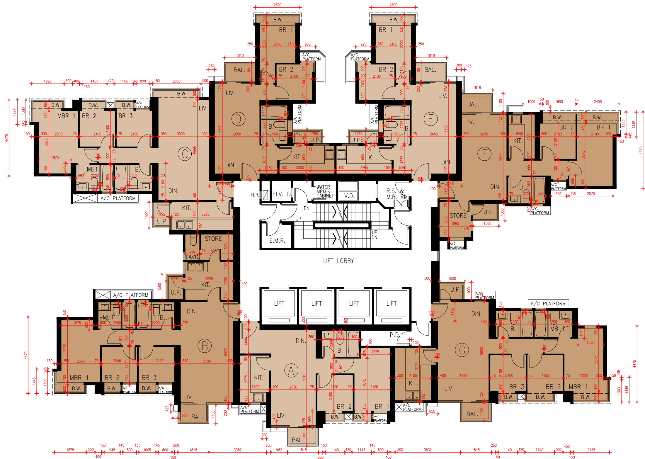
Tower 10 25/F - 33/F & 35/F - 42/F Floor Plan 第10座25樓至33樓及35樓至42樓樓面平面圖
