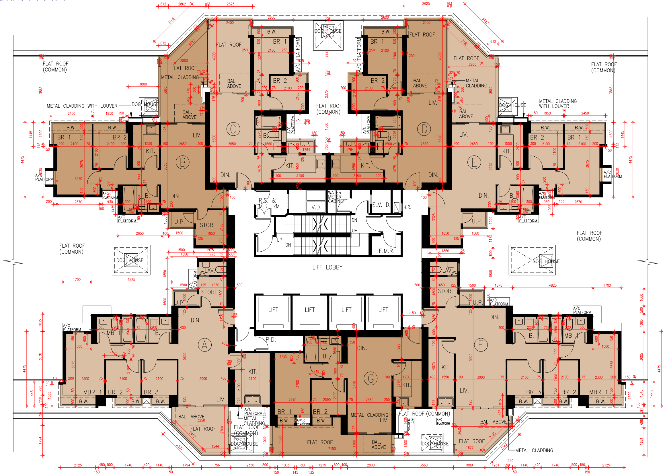
Tower 9 6/F Floor Plan 第9座6樓樓面平面圖
