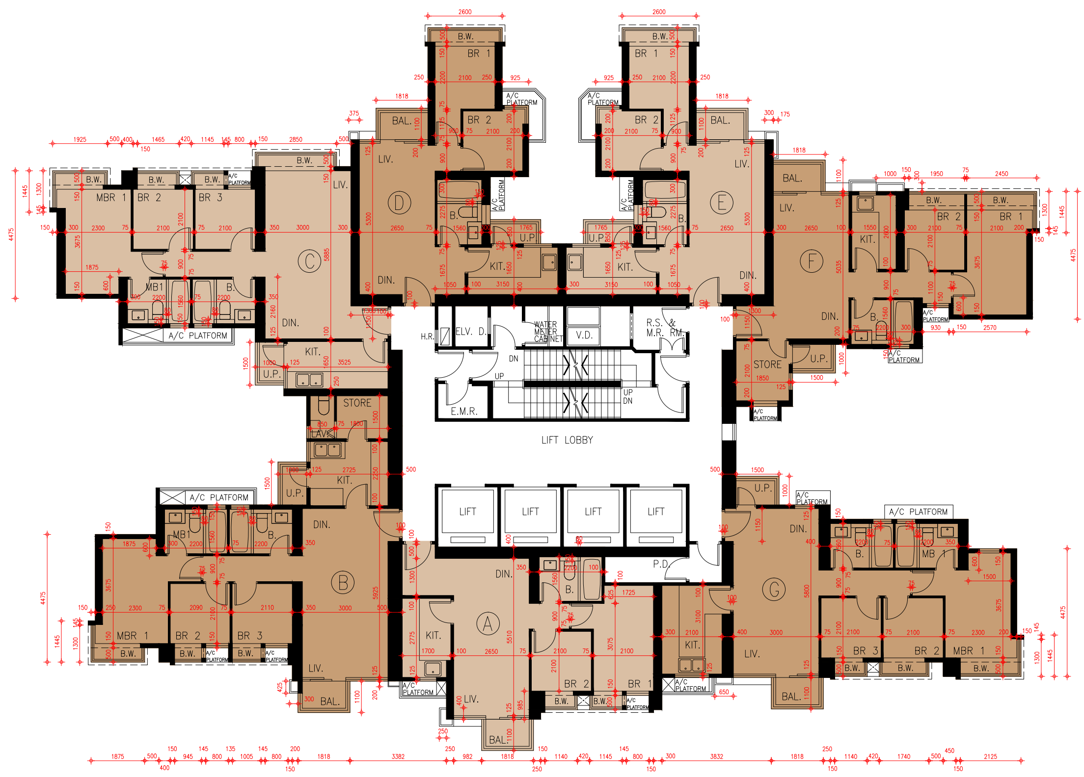
Tower 10 7/F - 13/F & 15/F - 21/F Floor Plan 第10座7樓至13樓及15樓至21樓樓面平面圖
