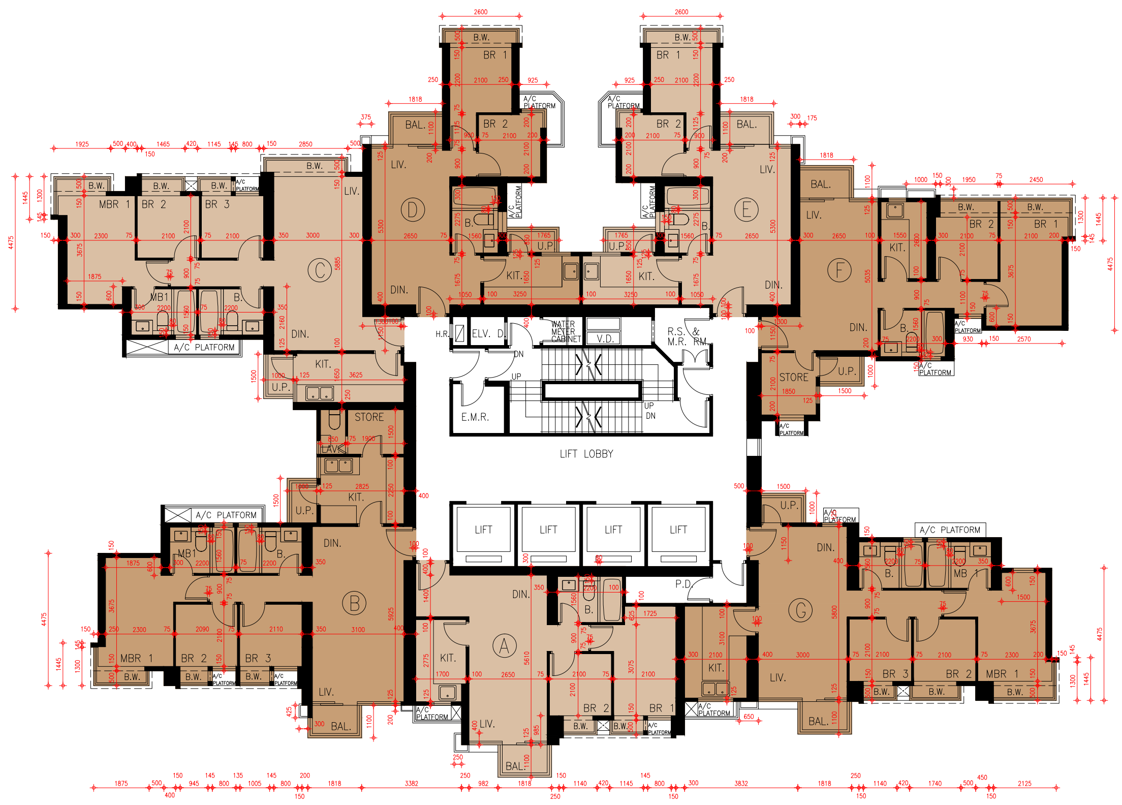
Tower 10 45/F - 48/F Floor Plan 第10座45樓至48樓樓面平面圖
