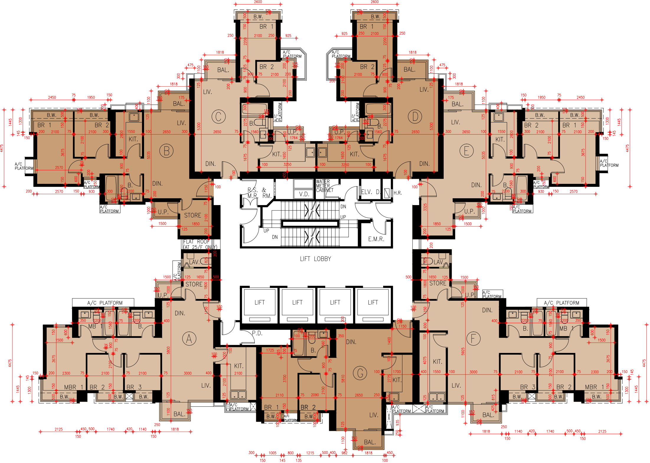
第9座25樓至33樓及35樓至42樓樓面平面圖
