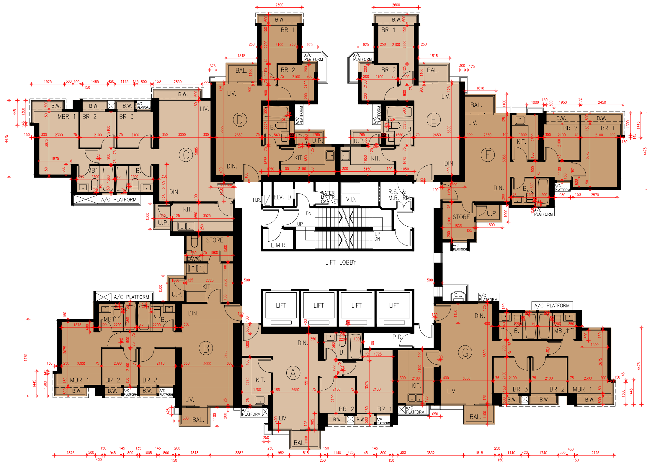
Tower 10 22/F Floor Plan 第10座22樓樓面平面圖
