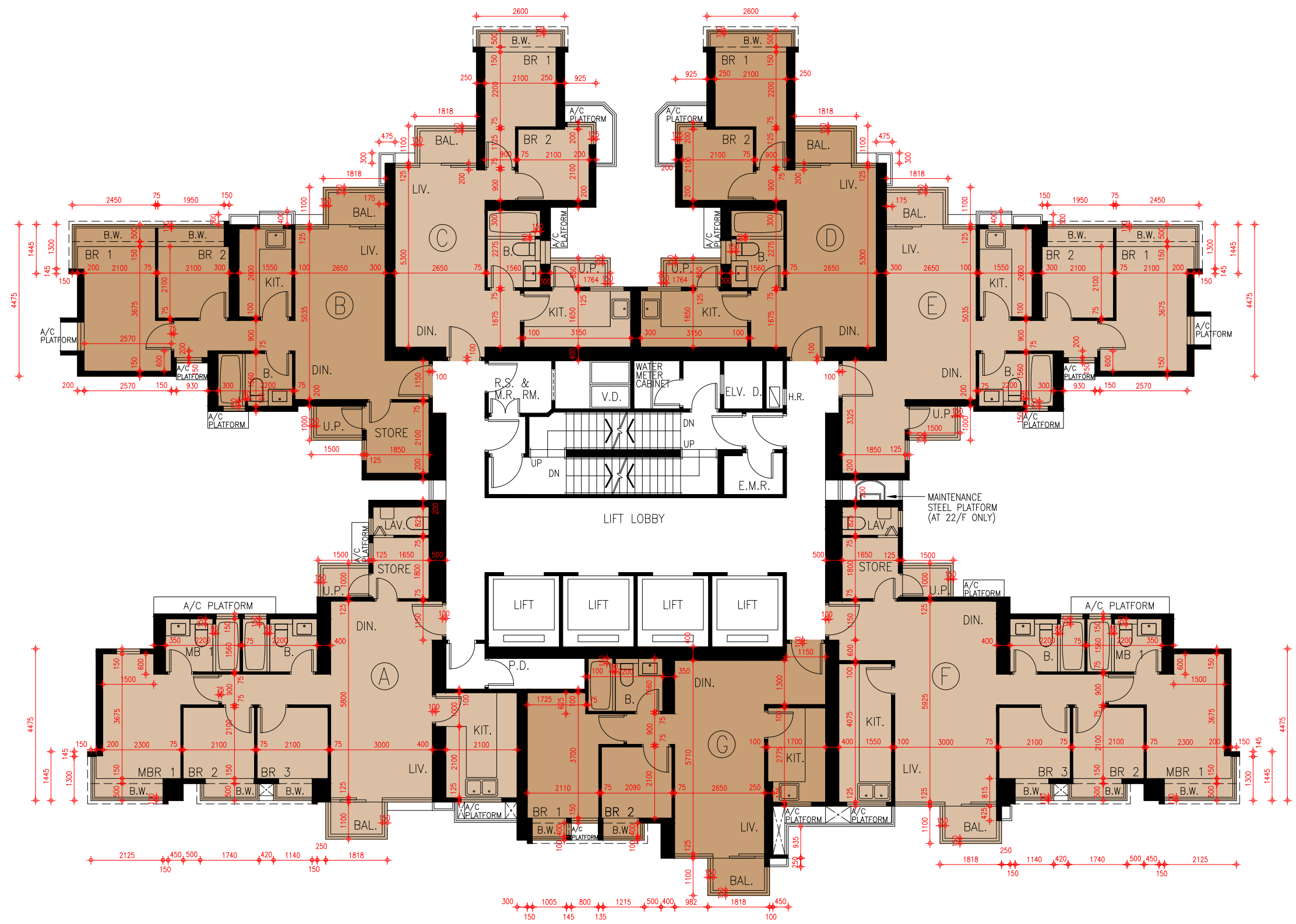
Tower 9 7/F - 13/F & 15/F - 22/F Floor Plan 第9座7樓至13樓及15樓至22樓樓面平面圖
