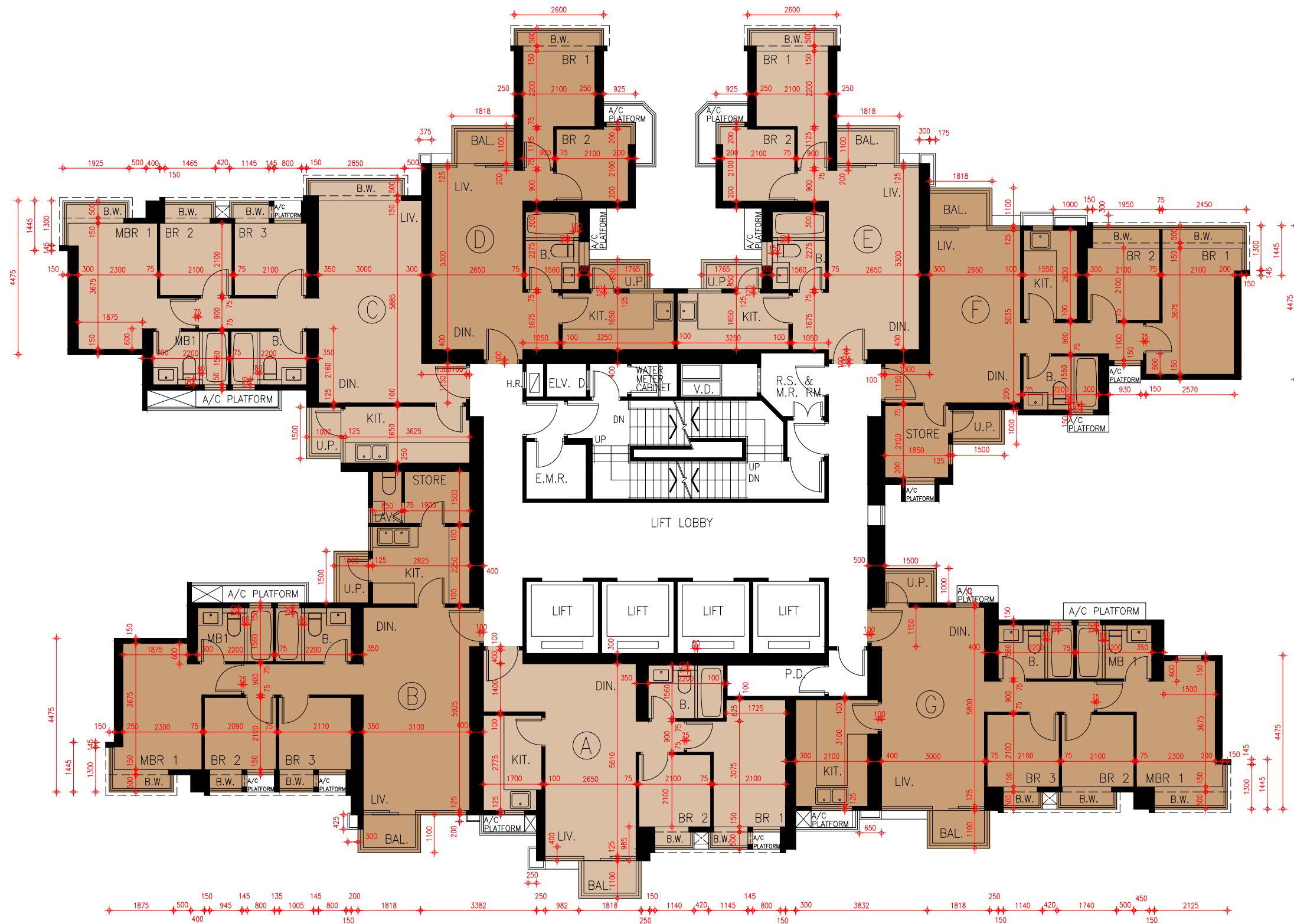
Tower 10 43/F Floor Plan 第10座43樓樓面平面圖
