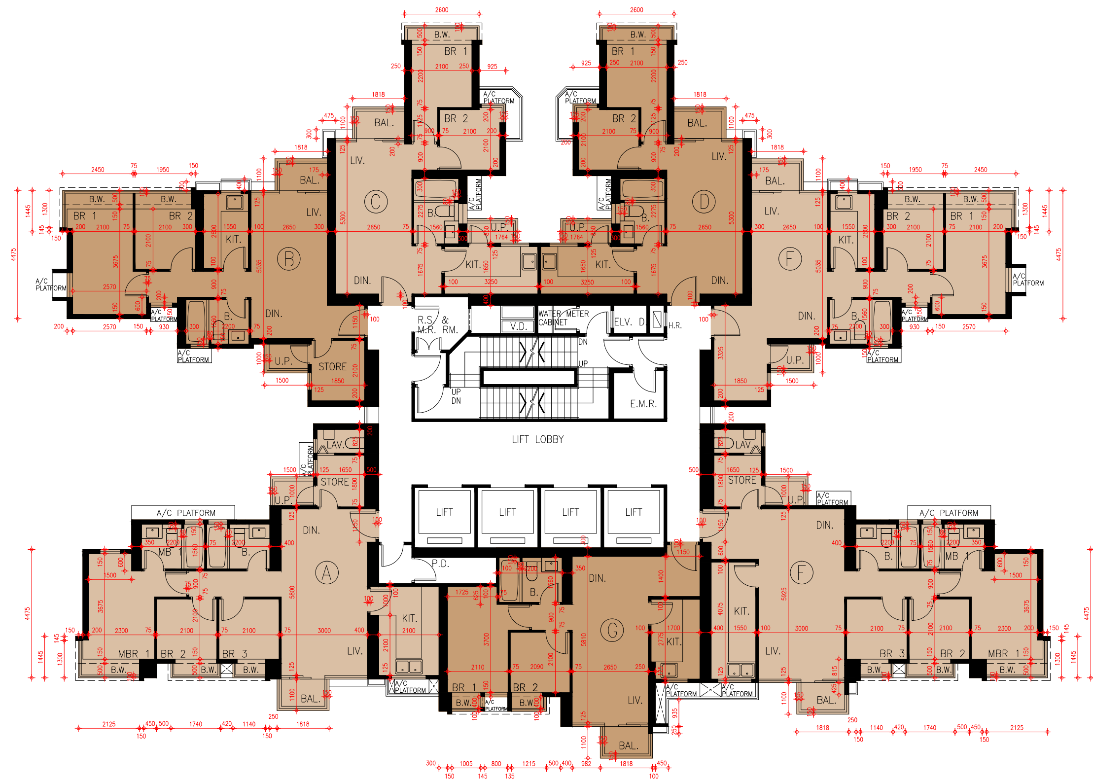
Tower 9 45/F - 48/F Floor Plan 第9座45樓至48樓樓面平面圖
