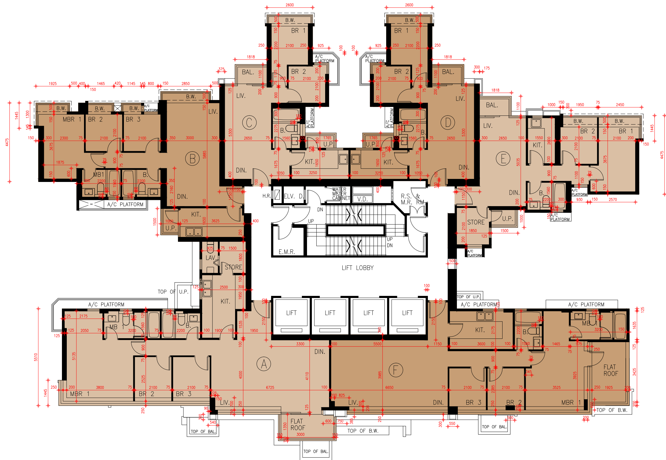
Tower 10 49/F Floor Plan 第10座49樓樓面平面圖
