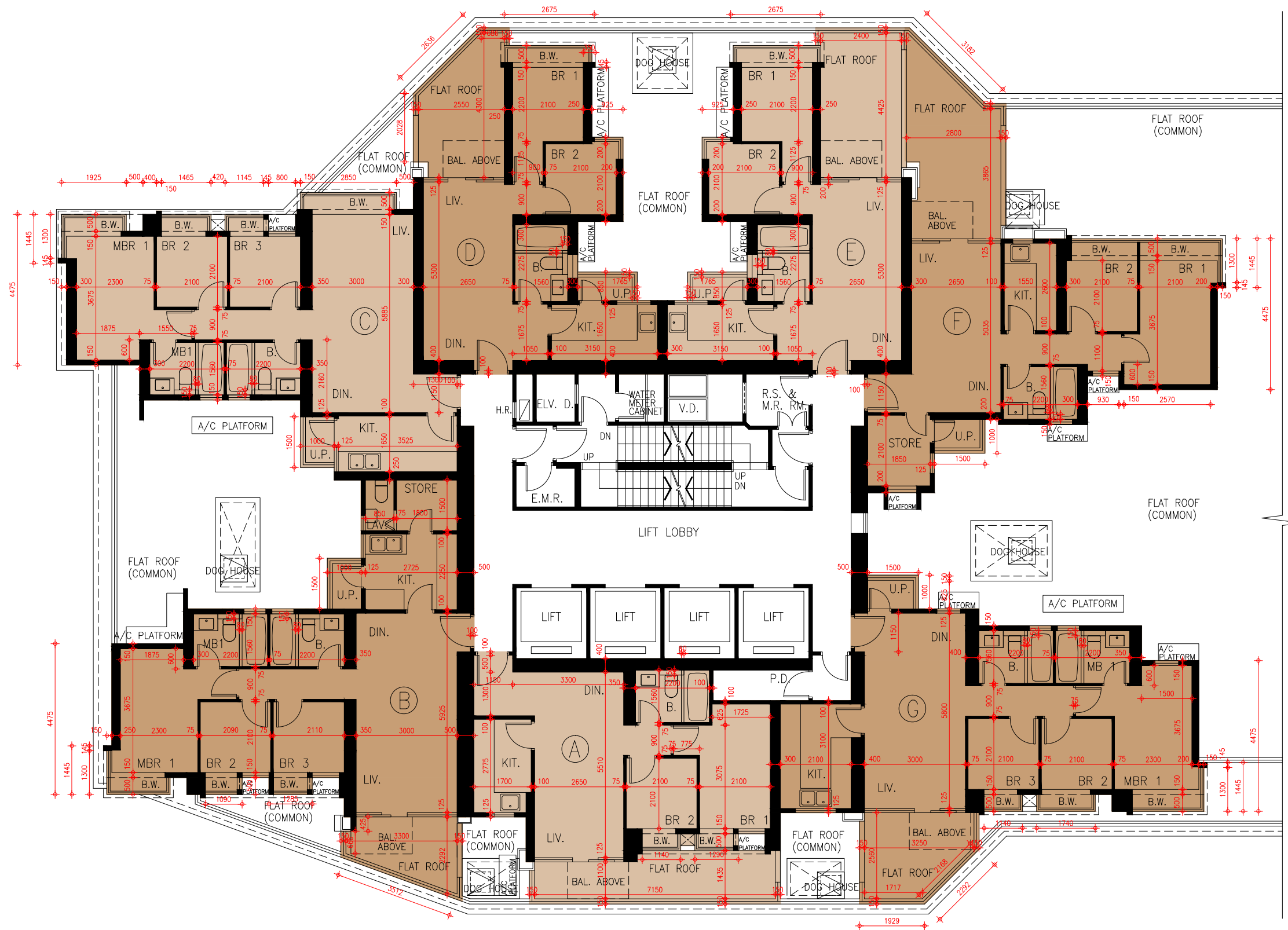
Tower 10 6/F Floor Plan 第10座6樓樓面平面圖
